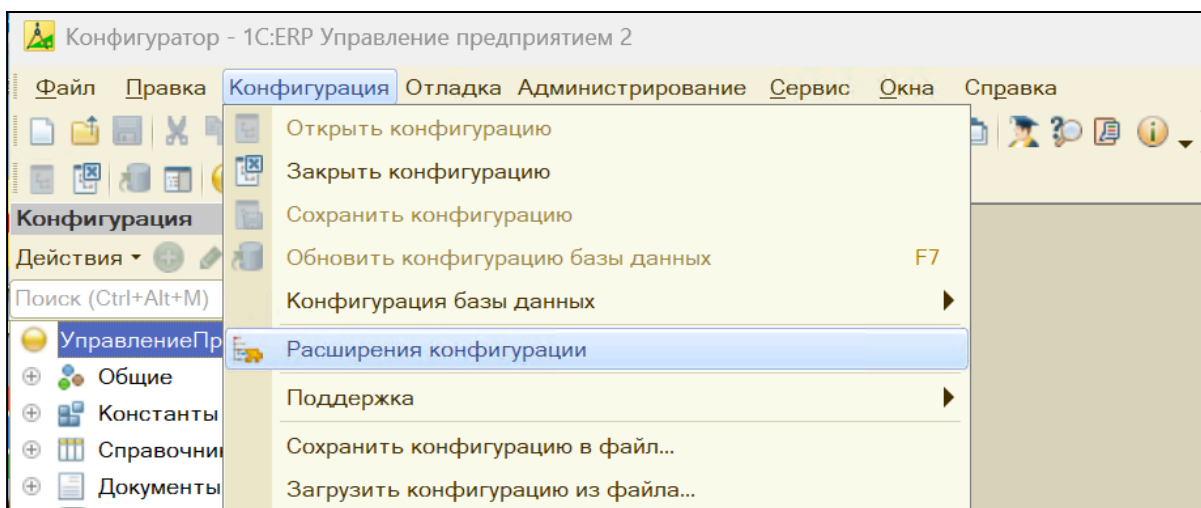
Рис. 3. Расширение конфигурации
