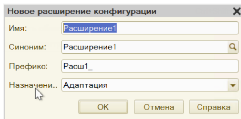
Рис. 5. Новое расширение
