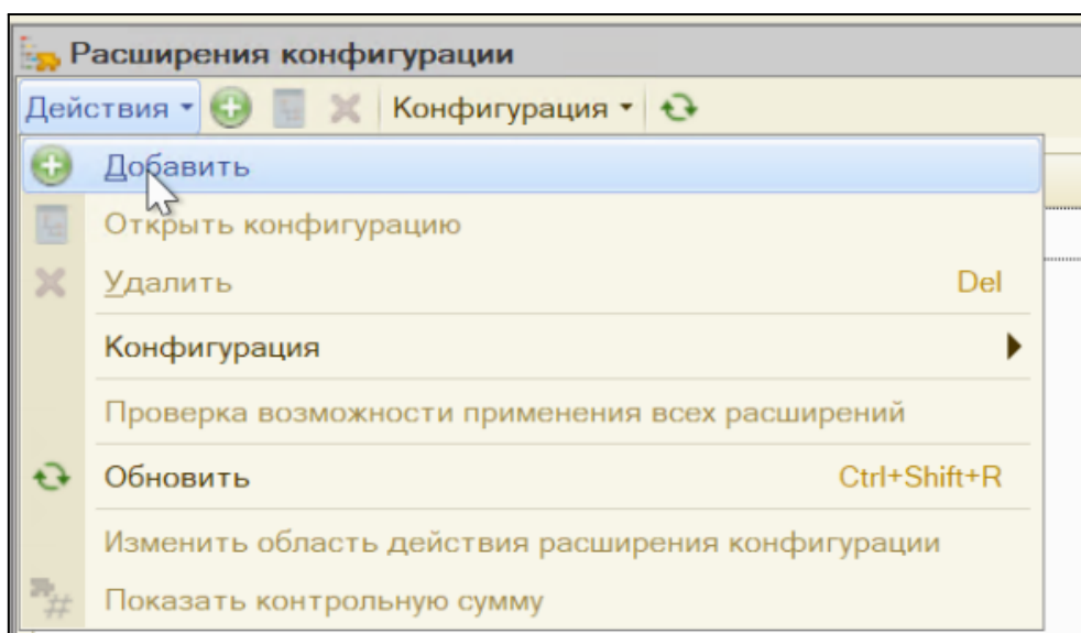
Рис. 4. Добавление расширения
