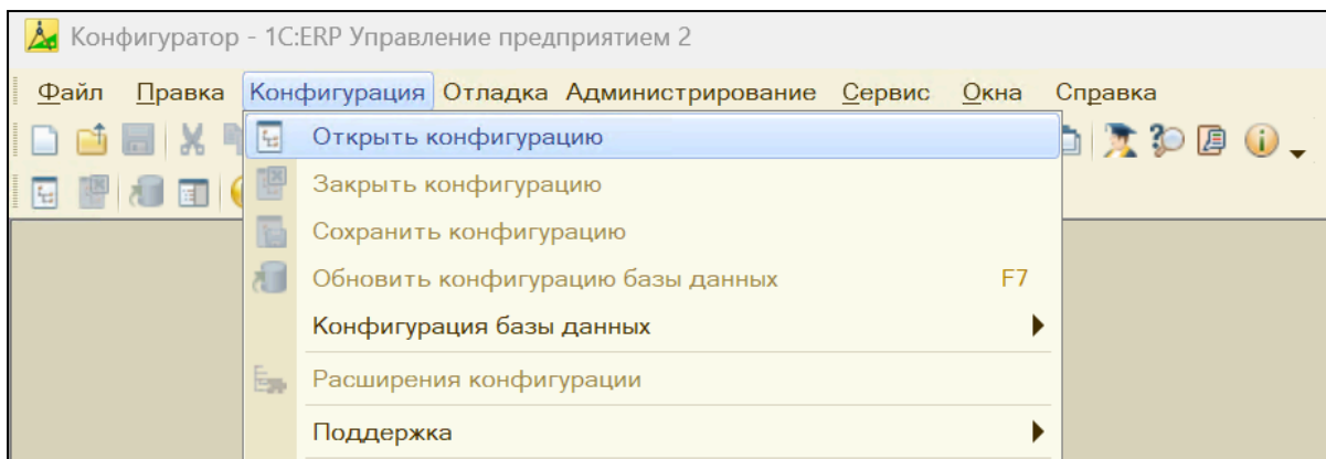
Рис. 2. Открытие конфигурации
