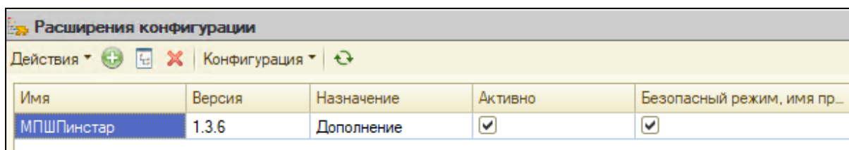
Рис. 11. Установленное расширение
